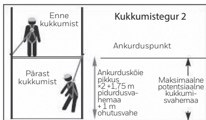
Joonis 3: minimaalne töötamiskõrgus
