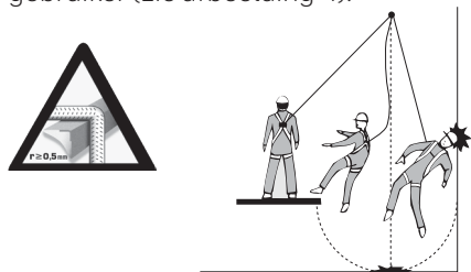
Afbeelding 4: slingerrisico
