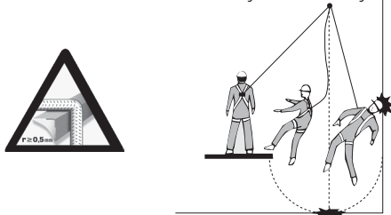
Joonis 4: kiikumise oht
