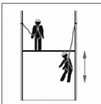
Facteur de chute 1
