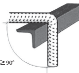
Figur 5: kantvinkel på iber eller lika med 90 grader tillåten användning.
