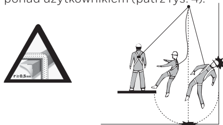
Rysunek 4: ryzyko kołysania
