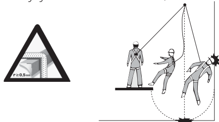
Kuva 4: Heilahdusvaara
