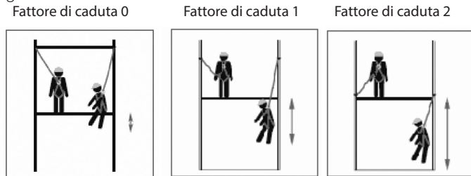
Figura 2: confronto dei fattori di caduta prima e dopo una caduta.
