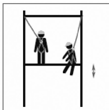
0 kritimo faktorius
