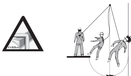
Figura 4: effetto pendolo
