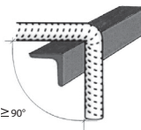
Kuva 5: Reunan kulma 90 astetta tai enemmän = käyttö luullinen
