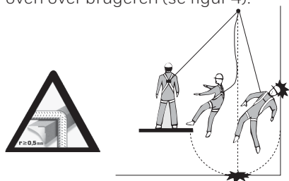
Figur 4: Svingfaktoren
