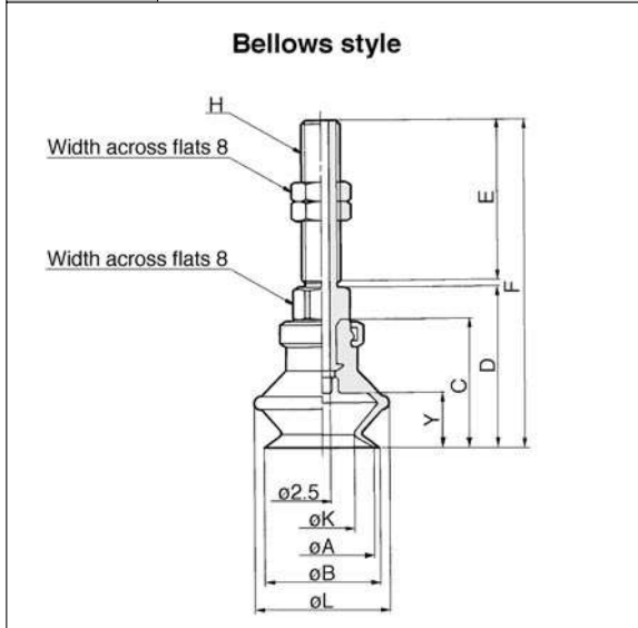
Pad Diameters ø10, ø13, ø16
