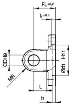
Mounting style (D)
