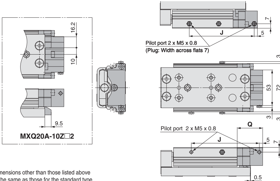
Dimensions
