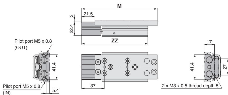
Dimensions
