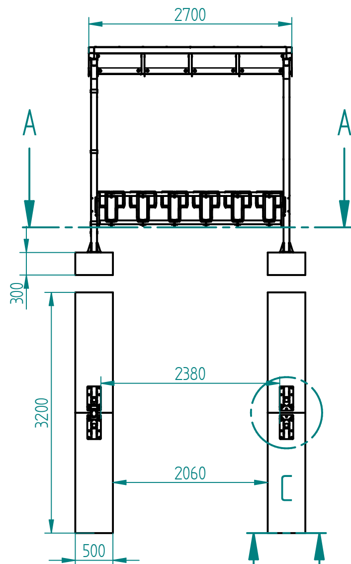
SECTION A-A
