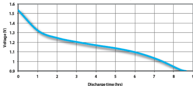
Portable lighting 4m/h 8h/d 3,3 ohm end 0,9V
