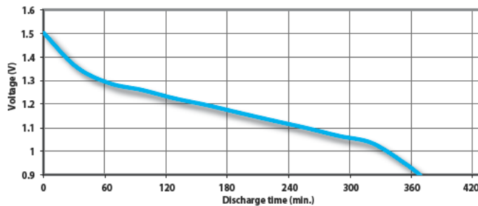
Portable lighting 4m/h 8h/d 3,3 ohm end 0,9V
